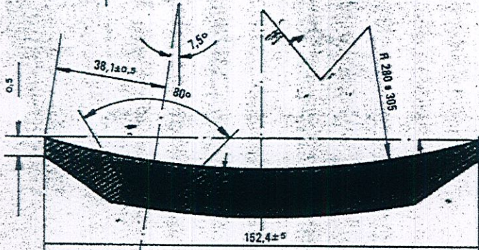
SECCION A - B SECTION A - B
